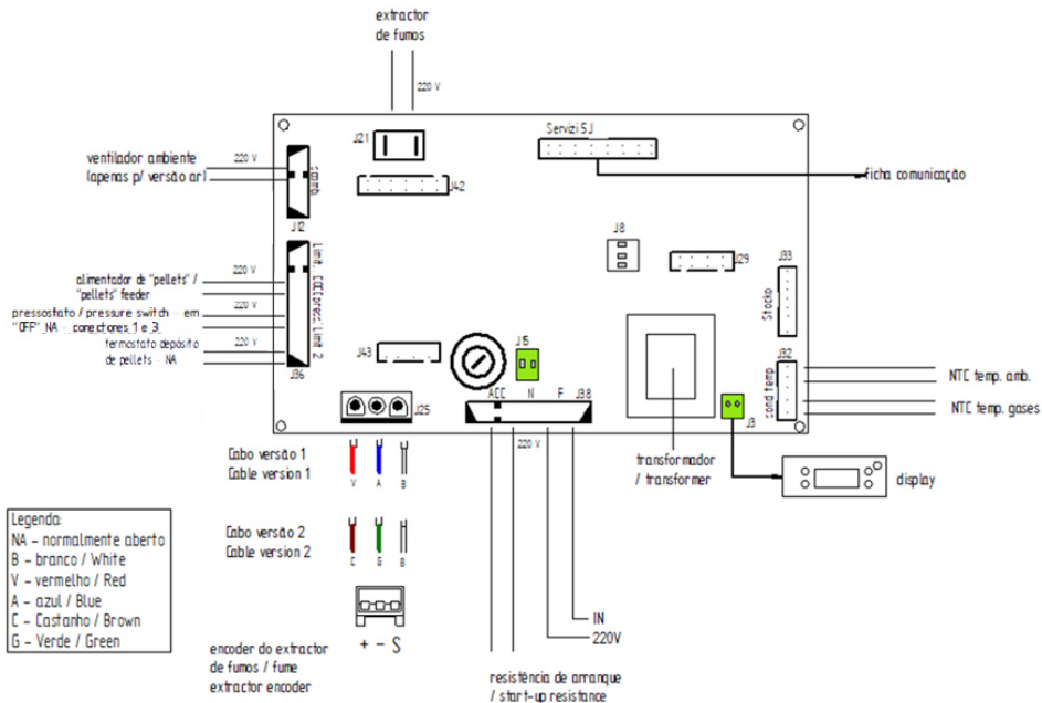
Figura 35 – Esquema elétrico Salamandra K50 (Europa)
